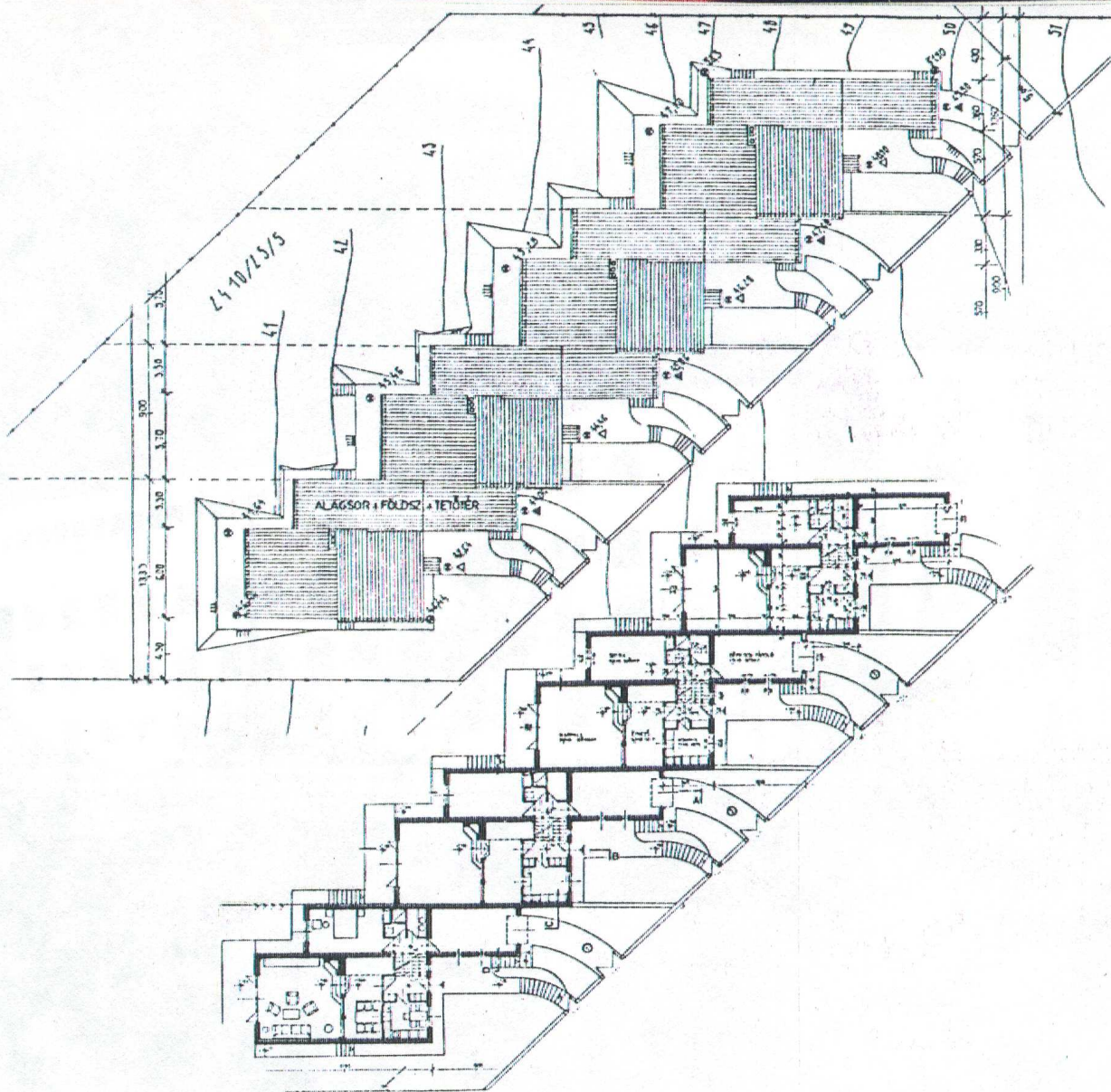
Budakeszi - Barackvirág út - Négylakásos társasház (1984)
